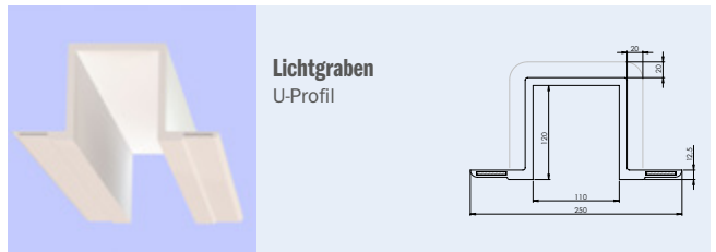
Lichtgraben U-Profil
