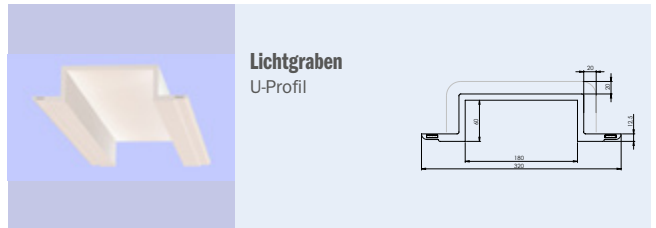
Lichtgraben U-Profil
