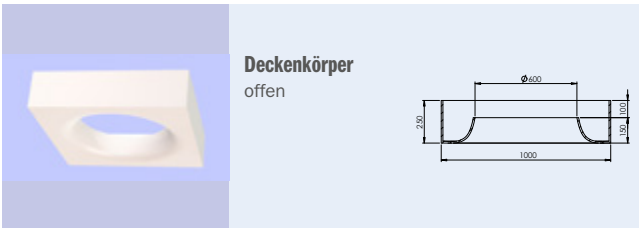
Deckenkörper mit Aussparung
