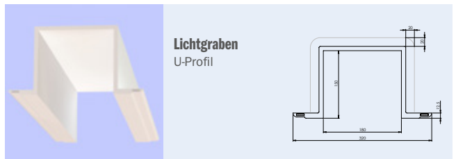
Lichtgraben incl. Auflegewinkel
