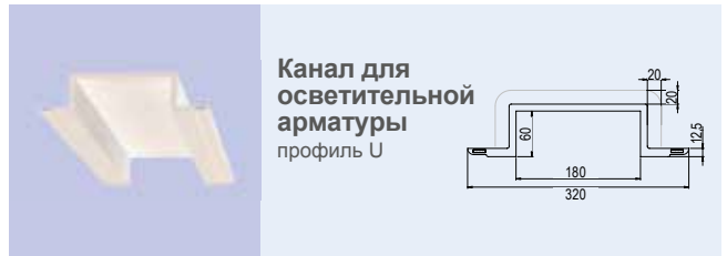
Канал для осветительной арматуры профиль U
