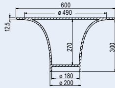
Воронка вогнутая
