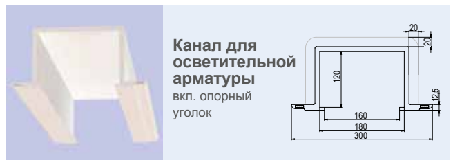
Канал для осветительной арматуры вкл. опорный уголок
